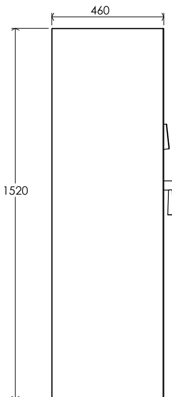
VISTA LATERAL
