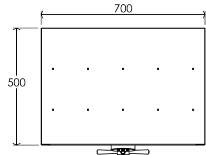
VISTA SUPERIOR
